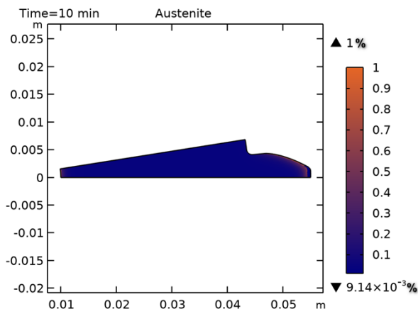
Hình 3. Tỷ phần Austenit còn dư
