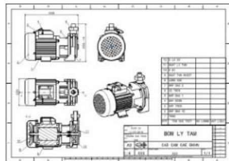
Hình 1. Bản vẽ lắp bơm ly tâm {figure}
